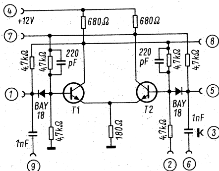
Bild 1. Schaltung eines Flipflop
