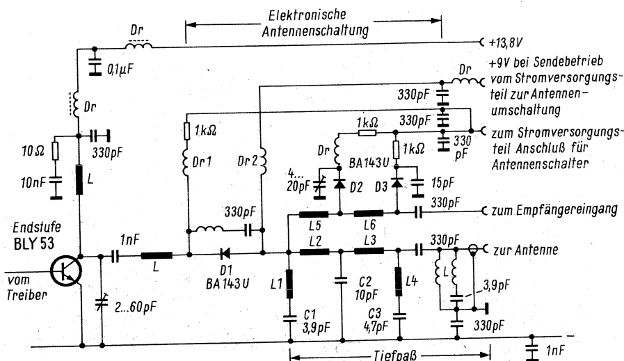
Bild 5. Elektronische Antennenumschaltung
