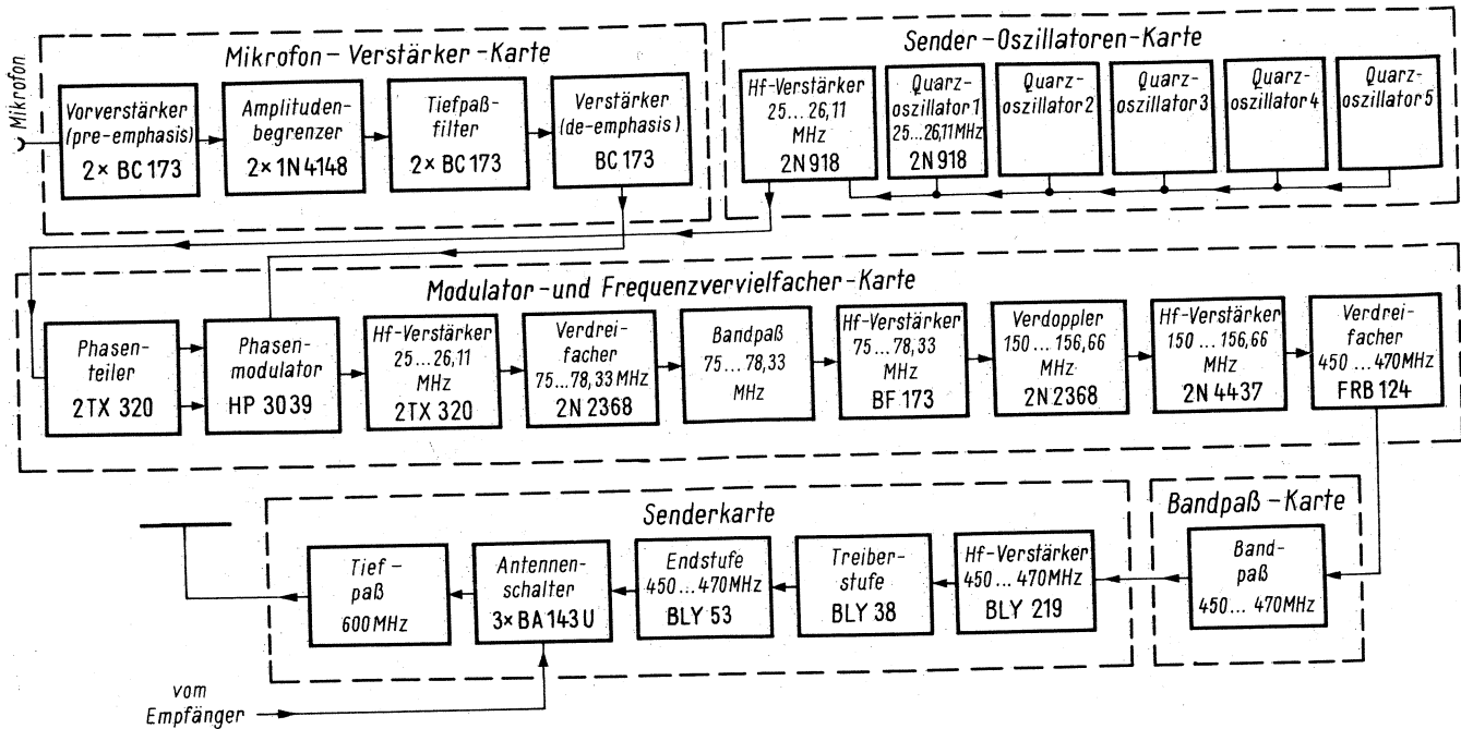
Bild 4. Blockschaltbild vom Senderteil
