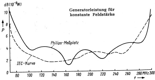
◀ Bild 7 Vergleich der gemessenen Eichkurve mit der IEC-Kurve im VHF-Bereich
