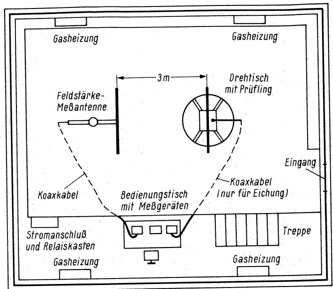
Bild 2 ▶ Schematische Aufsicht auf den Meßplatz
