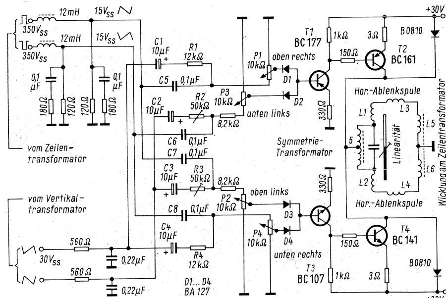
Bild 10. Durch Treiberstufen erweiterte Schaltung nach Bild 8
