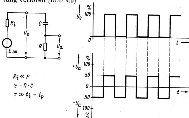
Bild 4.4. RC-Hochpaß; \tau \gg t_i = t_p ; diese Schaltung gewinnt aus einer Rechteckimpulsfolge eine Rechteckwechselfspannung
