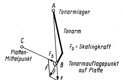
Bild 1. Entstehung der Skatingkraft mit Kräfteparallelogramm
