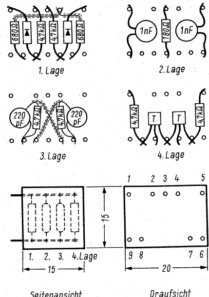
Bild 3. So werden die Bauelemente lagenweise geschichtet
