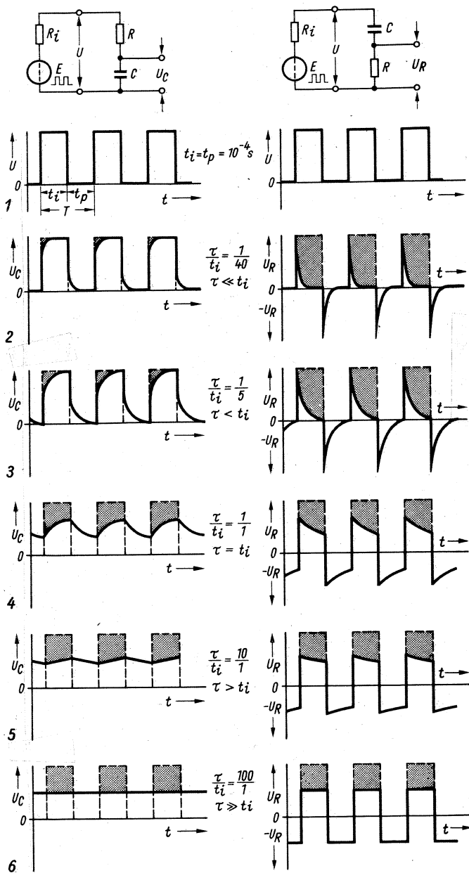
Bild 4.7. Impulsverformung durch RC-Glieder
