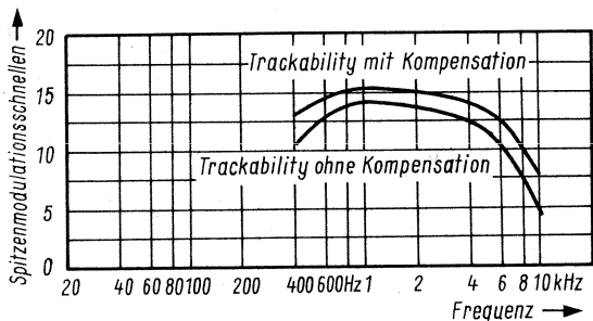
Bild 10. Trackability mit und ohne Skatingkraft-Kompensation
