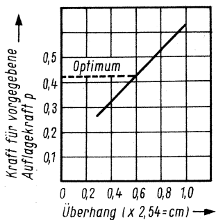
Bild 9. Änderung der Skatingkraftkompensation als Funktion des Überhangs im Shure-SME-Tonarm
