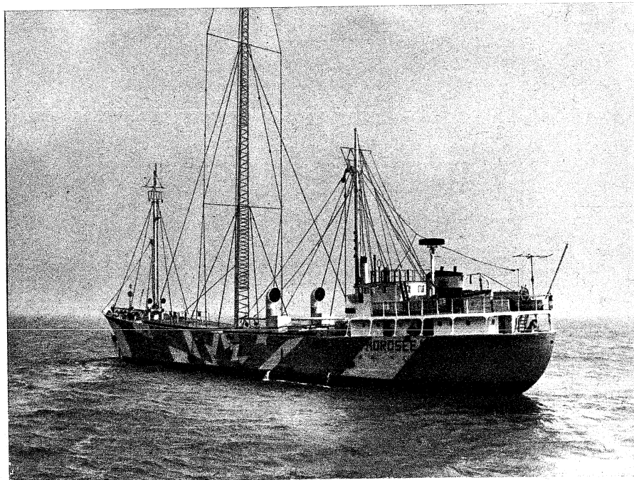
Der ehemalige Küstenfrachter wurde Mebo II genannt (Mebo I ist ein dazu gehöriges Versorgungsschiff). Das Schiff trägt jetzt vier Sender und vier Antennenanlagen. Deutlich ist die enge Nachbarschaft der einzelnen Antennen untereinander zu erkennen. Eine gegenseitige Beeinflussung ist daher praktisch nicht auszuschließen (Aufnahme: E. Jacob)
