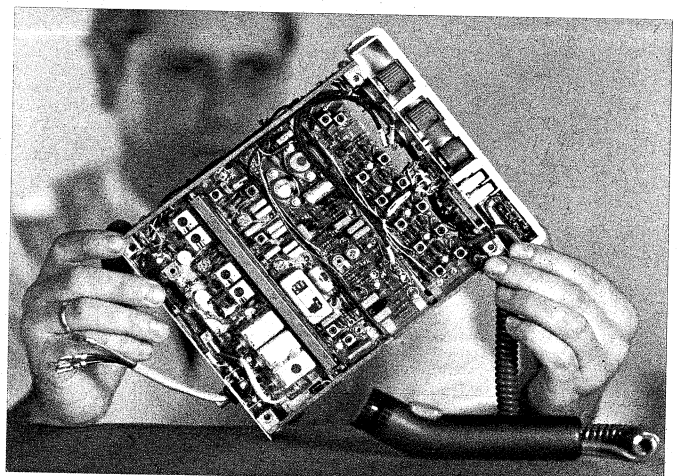
Bild 3. Unterseite mit dem Empfängerteil (zugleich Titelbild)
