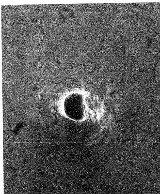
Bild 11. Einseitig abgeschliffener Diamantabstaststift nach Lebensdauer-test ohne Kompensation der Skatingkraft
