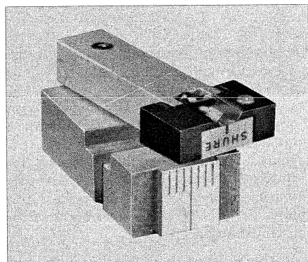
Bild 3. Der Skatingkraft-Detektor
