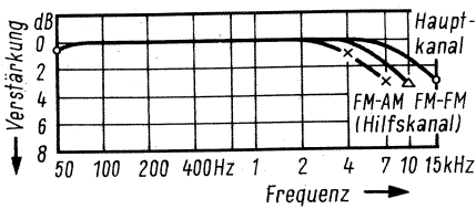
Bild 2. Amplituden-Frequenzgang des FM-FM- und des FM-AM-SSB-Multiplexverfahrens für den Haupt- und den Hilfskanal
