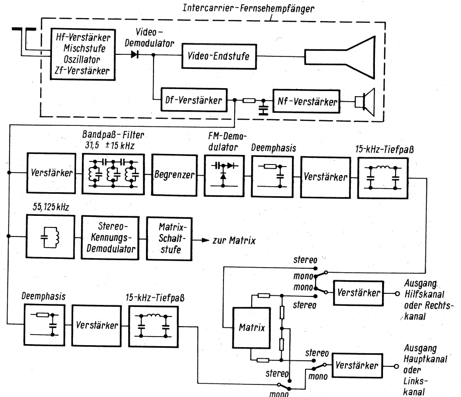
Bild 9. Anschlußschema und grundsätzlicher Aufbau eines Empfangsadapters nach dem FM-FM-System zum Nachrüsten eines Intercarriempfängers
