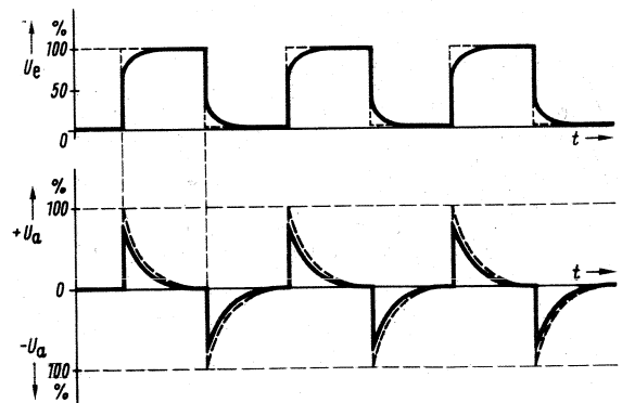
Bild 4.9. RC-Differenzglied; Einfluß des Innenwiderstandes im Pulsspannungserzeuger auf den zeitlichen Verlauf der Größen U_e und U_a
