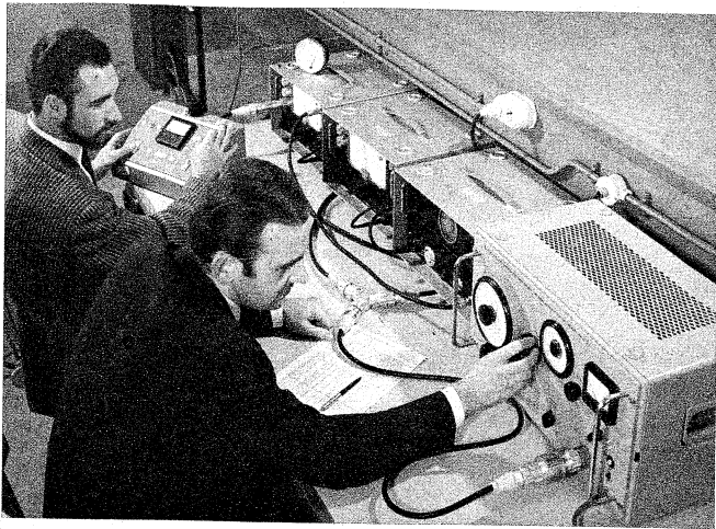
Bild 6 ▶ Zusammenstellung der Meß- und Eichantennen
