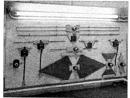
Bild 6 ▶ Zusammenstellung der Meß- und Eichantennen
