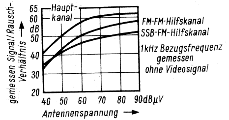
Bild 4. Signal/Rausch-Verhältnis als Funktion der Antennenspannung beim FM-FM- und FM-AM-SSB-Verfahren für den Haupt- und den Hilfskanal
