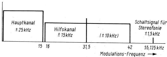
Bild 7. Frequenzbandverteilung des FM-FM-Verfahrens
