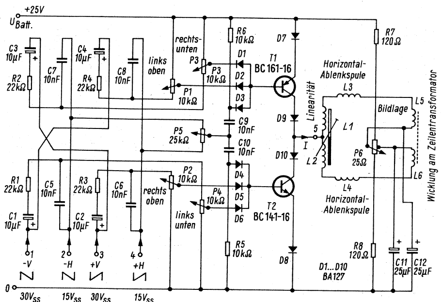
Bild 8. Prinzip der Eckenkonvergenzschaltung
