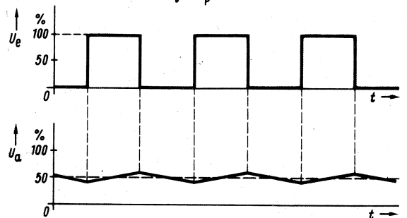
Bild 4.6. RC-Integrierglied; \tau = 5 \cdot t_i \tau = 5 \cdot t_p
