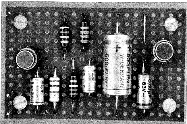
Bild 2. Aufbau und Platine des Mustergerätes
