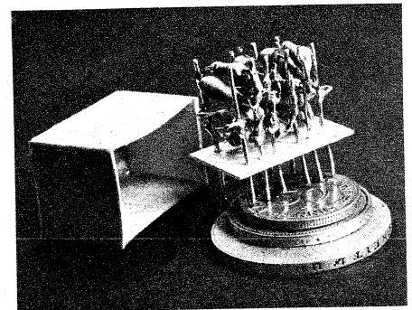
Bild 4. Noch nicht vergossener Modul mit abgenommener Schutzhaube (Aufnahme: Leutmayer)
